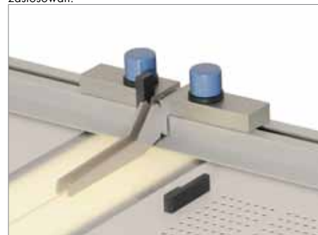
Szybko wymienne spacjiatory magnetyczne umożliwiają łatwiejszą niż dotychczas regulację odległości między tekturkami montażowymi a paskiem grzbietowym.
